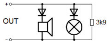
Fig. 1: Control de línea de dispositivo de señalización EN 54 con una resistencia RFL de 3,9 k \Omega
