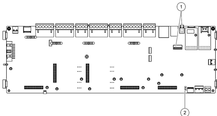
Figura 4: Los conectores USB y JP4 de la PCB de la central
