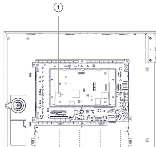
Figura 3: Ubicación del conector USB tipo A de la placa de la pantalla táctil
