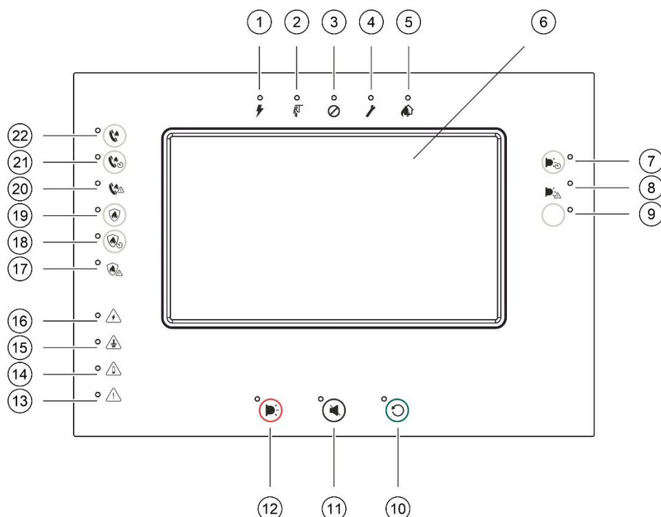
Figura 1: Interfaz de usuario (con controles de protección y enrutado de incendios)
