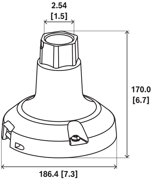
Fig. 1: Dimensiones en mm (pulg.) de NDA-7100-PIPE | NDA-7100-PIPEF
