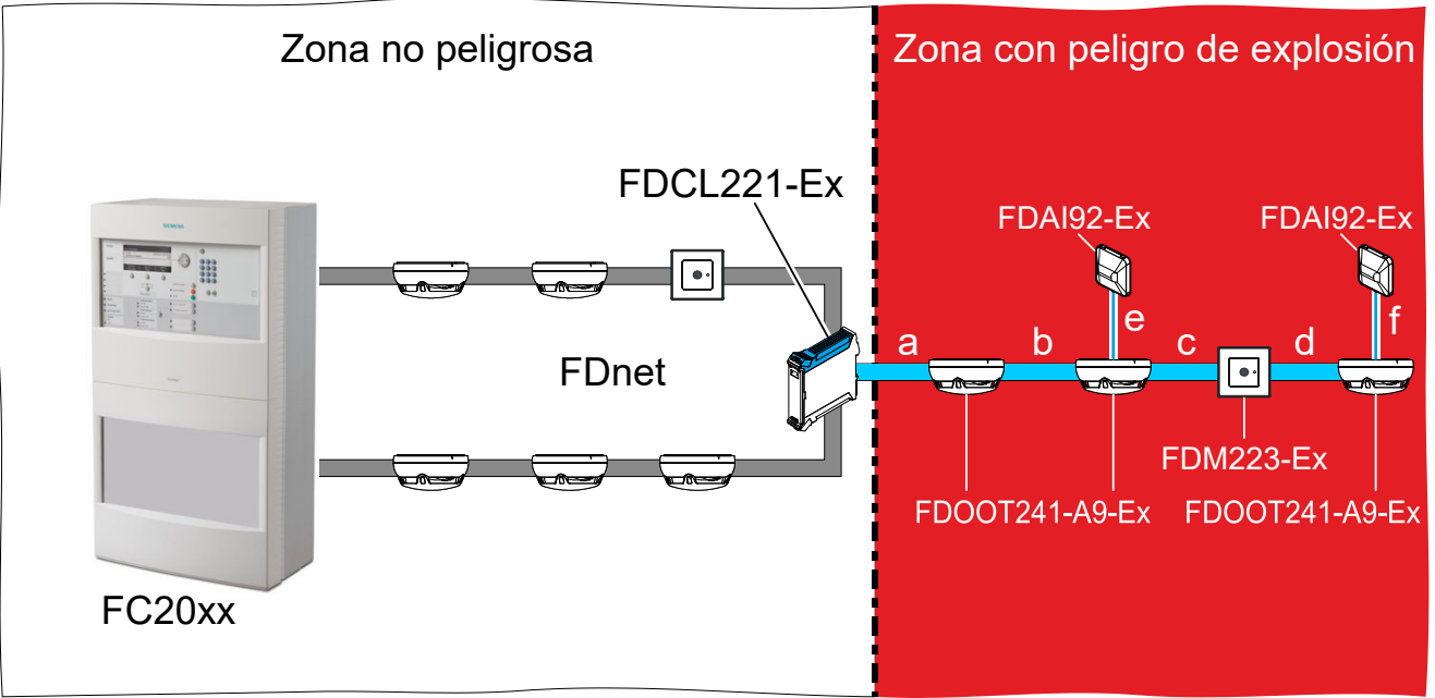
Fig. 12: Ejemplo de una instalación de detección de incendios Sinteso en una zona con riesgo de explosión
