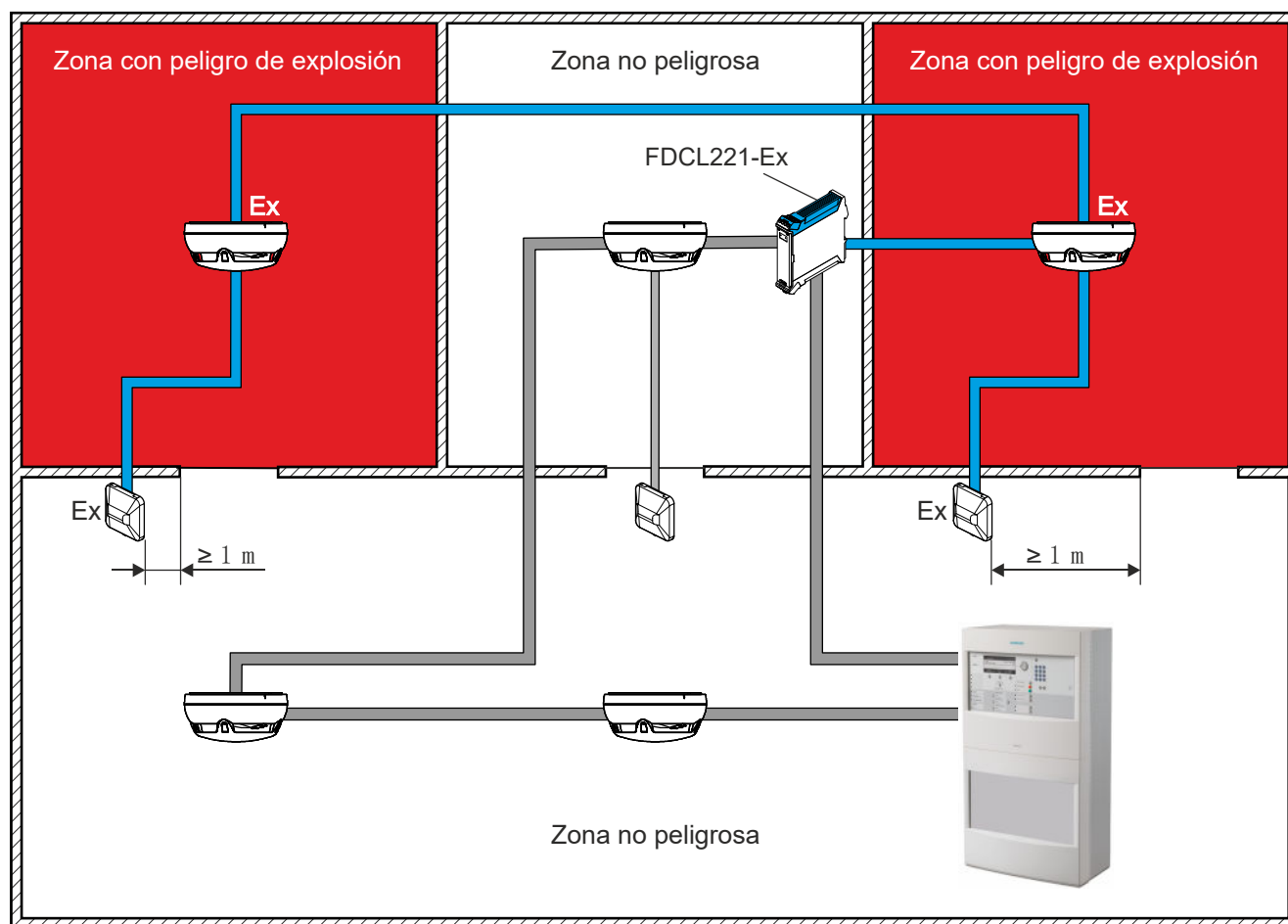
Fig. 10: Colocación de cables en zonas sin peligro de explosión
