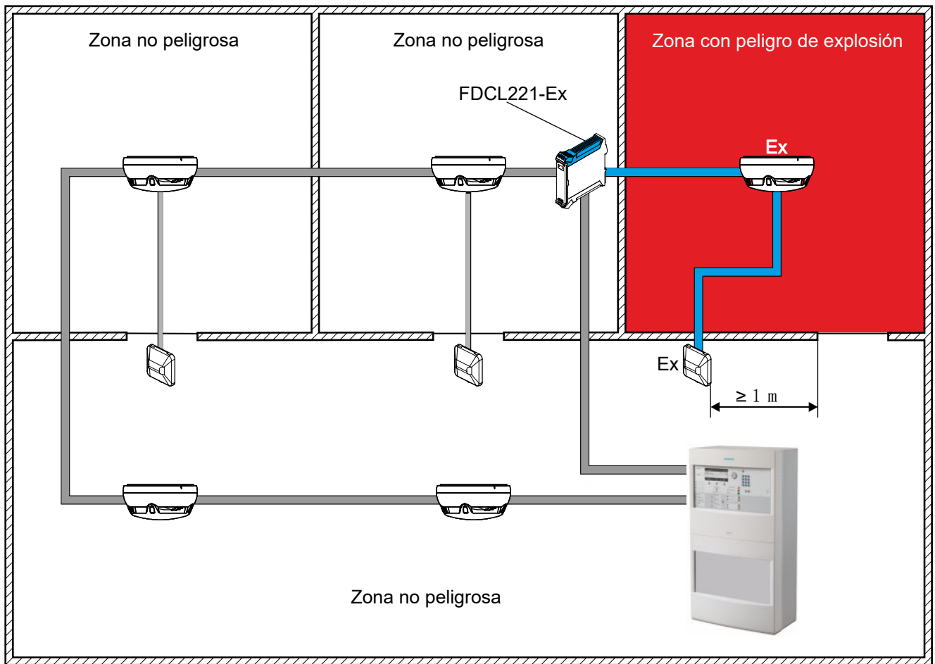
Fig. 9: Ejemplo de una instalación de detección de incendios en una zona con riesgo de explosión
