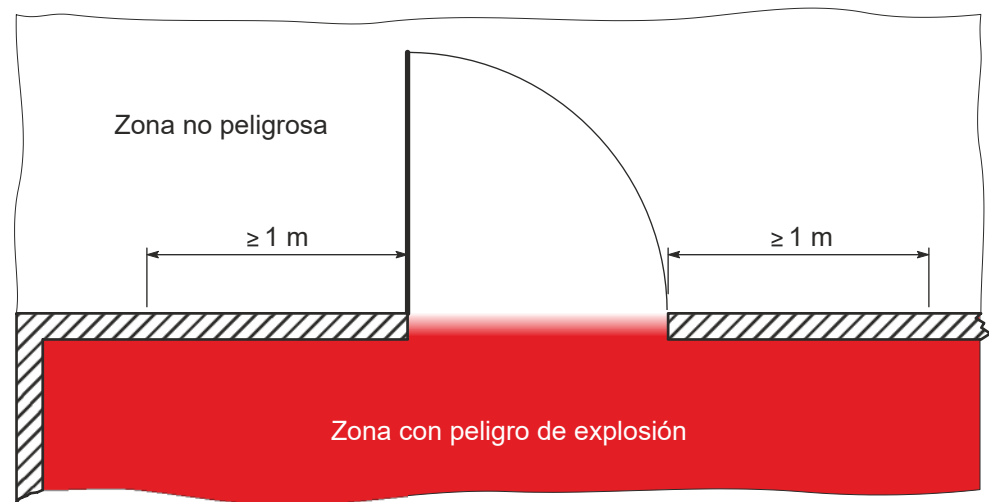
Fig. 6: Distancia de seguridad junto a huecos de paso y orificios de ventilación
