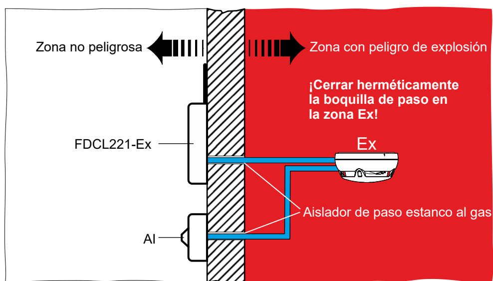
Fig. 11: Representación esquemática de la disposición habitual de un indicador de alarma externo
