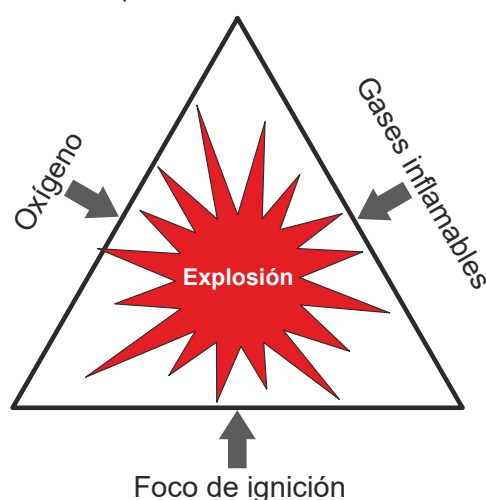
Fig. 1: Triángulo de explosión
