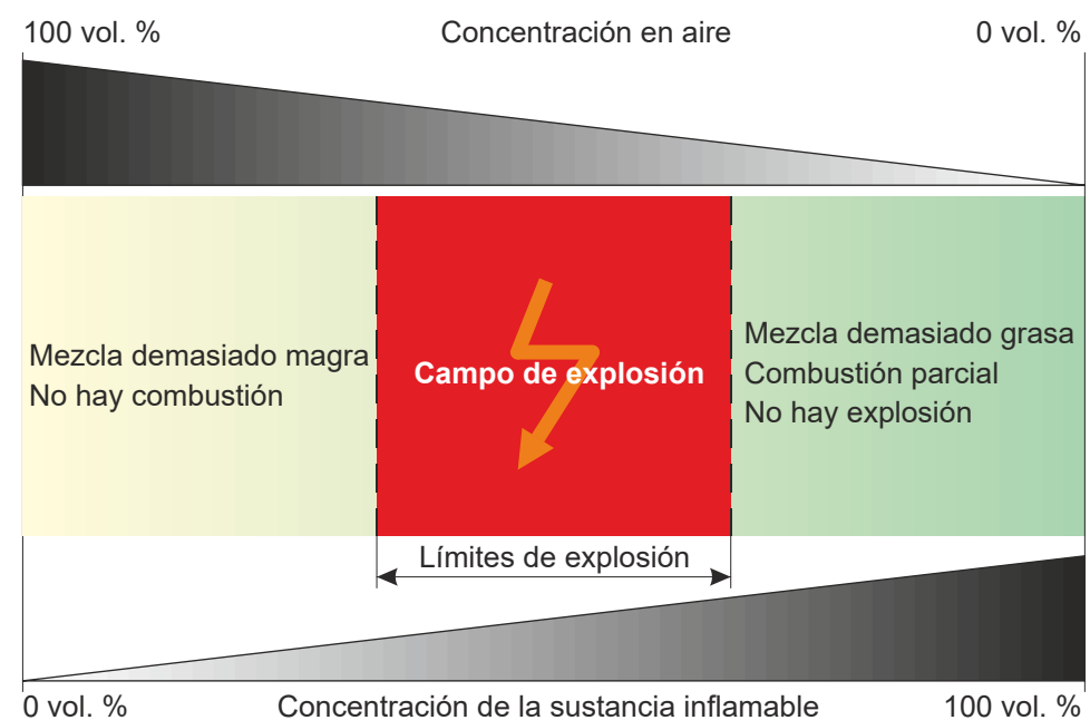
Fig. 2: Límites de explosión
