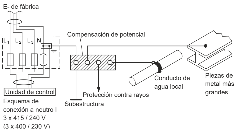
Fig. 7: Ejemplo de una puesta a tierra de conexión equipotencial
