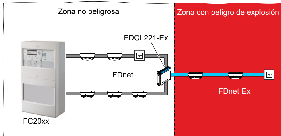
Fig. 4: Ejemplo de instalación de una instalación de detección de incendios FS20 en una zona Ex y en una zona sin peligro de explosión
