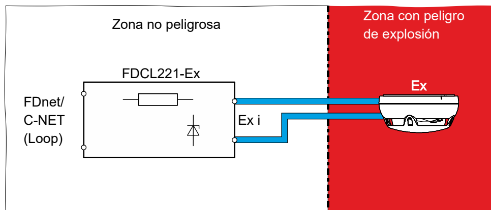
Fig. 8: Adaptador de línea (Ex) FDCL221-Ex
