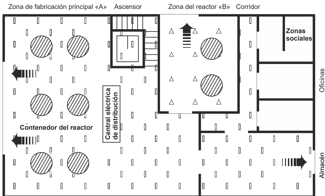
Fig. 3: Ejemplo de una distribución en zonas:
