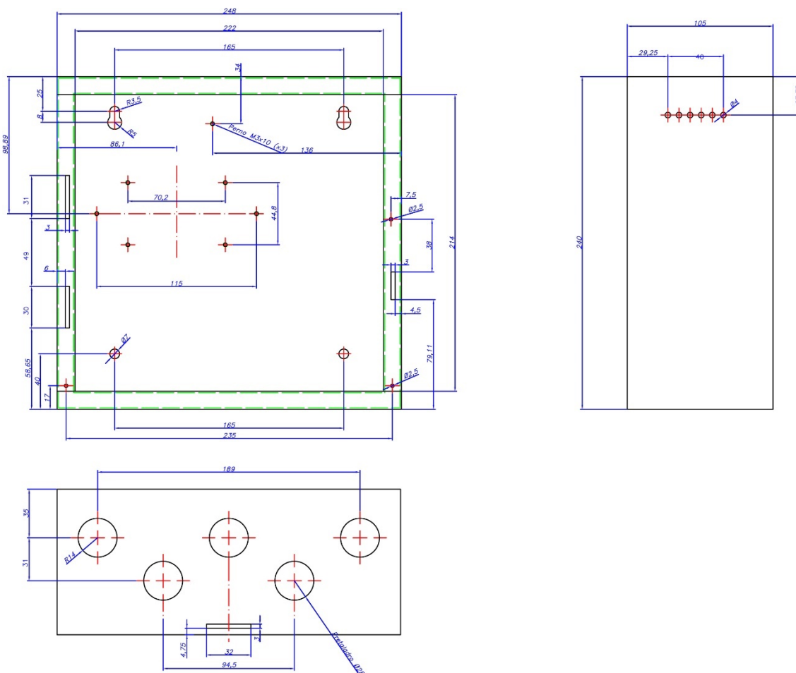
Figure 4: Dimensions coffre et porte de la centrale (mm).
