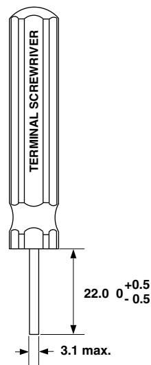
Fig. 2: Elaboración de una herramienta de desbloqueo 1- Extremo final perpendicular al mango
