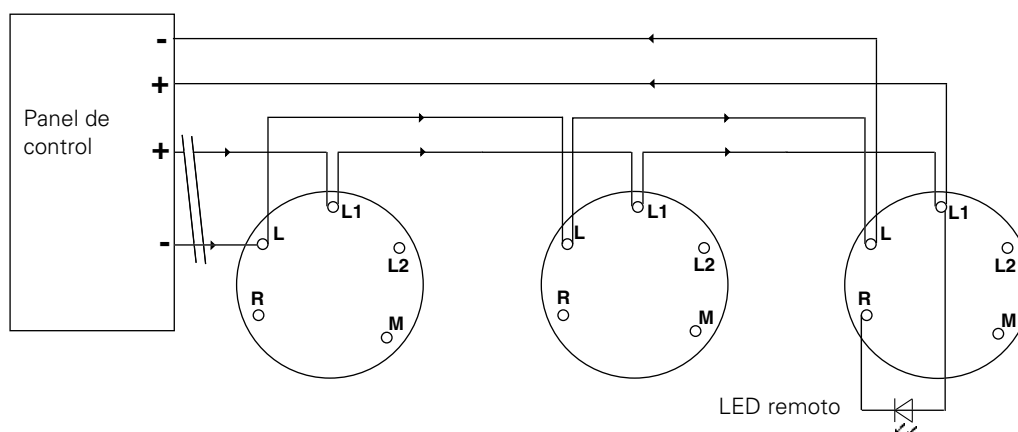
Fig. 5: Esquema de conexiones de implementación típica: 4B
