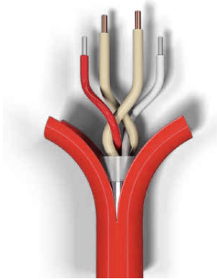
ProReact EN Analogue Sensor Cable
