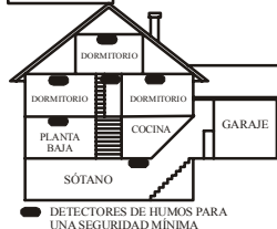
Figura 3: INSTALACIÓN DE LOS DETECTORES DE HUMOS EN RESIDENCIAS DE MÁS DE UNA PLANTA.
