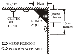
Figura 4: LUGARES RECOMENDADOS PARA LA INSTALACIÓN DE LOS DETECTORES DE HUMOS.
