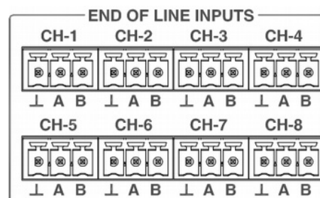
Ilustración 14: Entradas Terminadores de Línea de Altavoces
