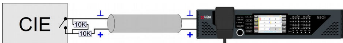
Ilustración 9: Conexión a ECI Supervisada
