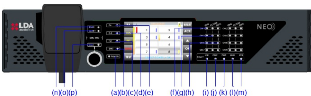
Ilustración 1: Indicadores
