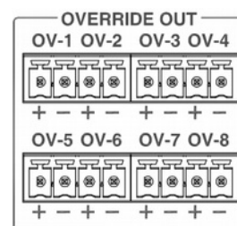
Ilustración 13: Salida Anulación Atenuadores
