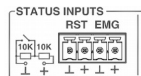
Ilustración 10: Entrada Activación de Emergencia General
