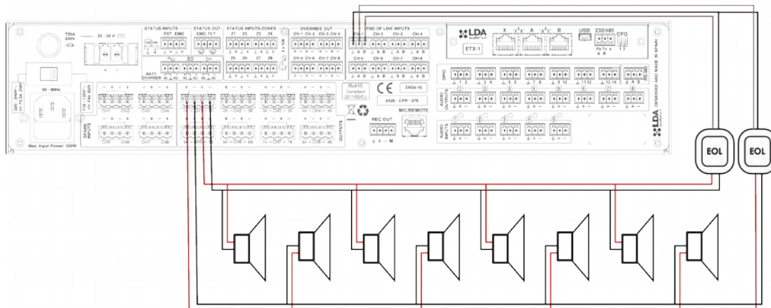
Ilustración 47: Líneas de Altavoces. Modo AB
