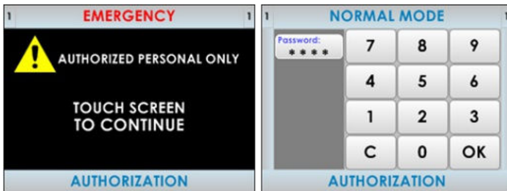
Ilustración 5: Tipos de Ventana de Control de Acceso
