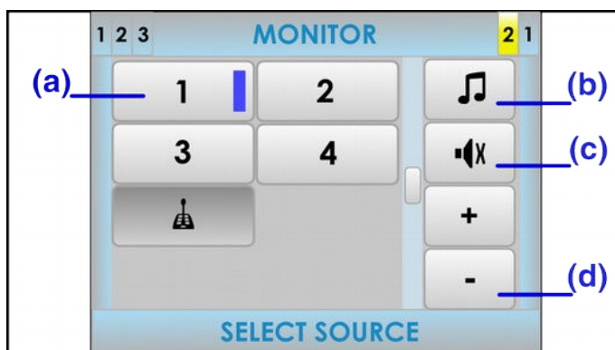
Ilustración 37: Ventana Monitor
