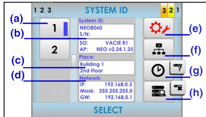
Ilustración 40: Ventana Sistema
