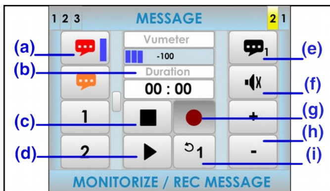
Ilustración 38: Ventana Mensajes
