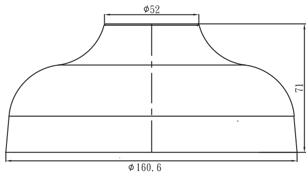
Placa accesoria para colgar NDA-4020-PIP Dimensiones en mm (pulgadas)
