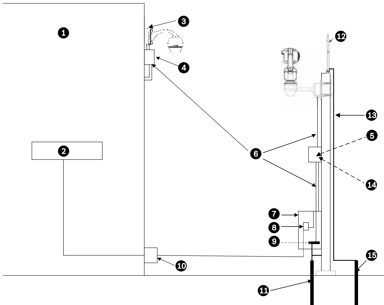
Figura 17.1: Corretta installazione all'esterno con corretta protezione da sovratensione/parafulmine
