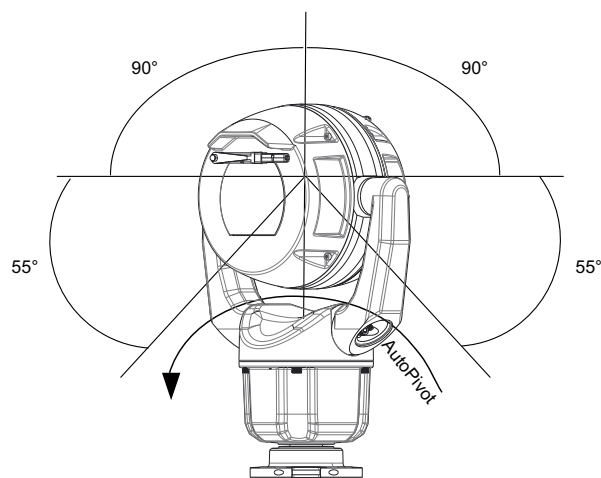
Figura 5.1: Intervallo di inclinazione, MIC IP ultra 7100i
