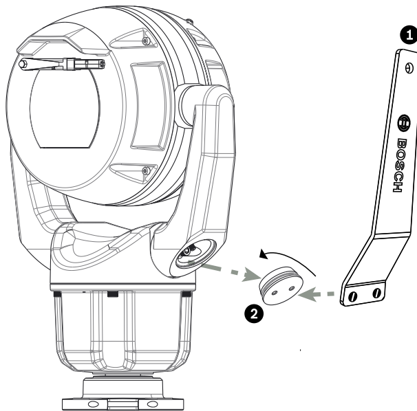
Figura 11.2: Rimuovere i cappucci della forcella con la chiave.
