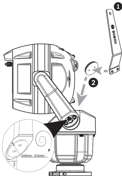
Figura 11.6: Fissare i cappucci della forcella.
