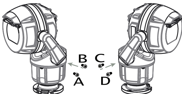
Figura 11.5: Inserire nuovamente le viti nei bracci della forcella nella seguente sequenza: ABCD.
