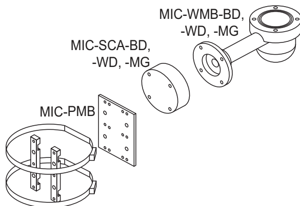
Figura 5.3: Configurazione tipica della staffa di montaggio su palo
