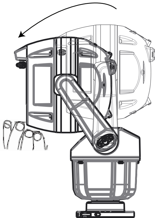
Figura 11.3: Inclinare la testa della telecamera.
