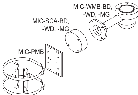
Figura 5.2: Configurazione tipica della staffa di montaggio su palo
