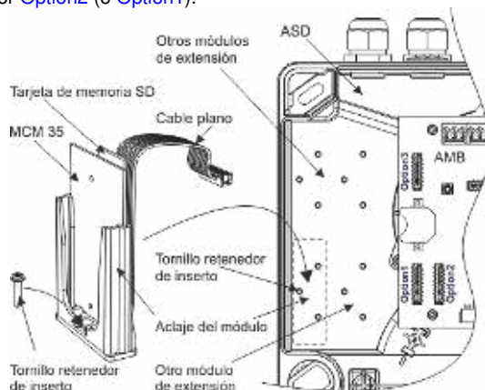
Fig. 2 Instalación del MCM 35
