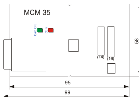
Fig. 4 MCM 35 dibujo dimensionado
