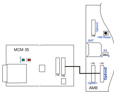
Fig. 3 Cableado del MCM 35
