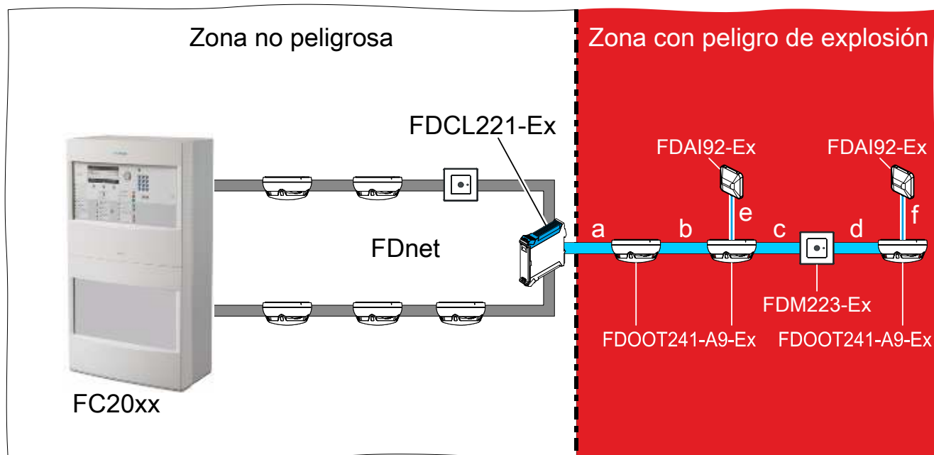
Figura 12: Ejemplo de una instalación de detección de incendios Sinteso planeada en una zona con peligro de explosión
