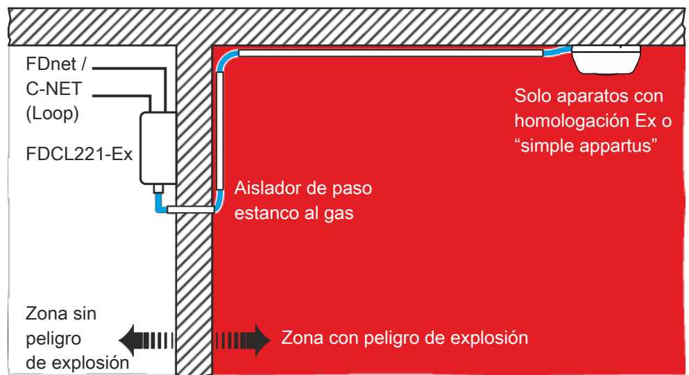
Figura 5: Ejemplo de una instalación en una zona con riesgo de explosión
