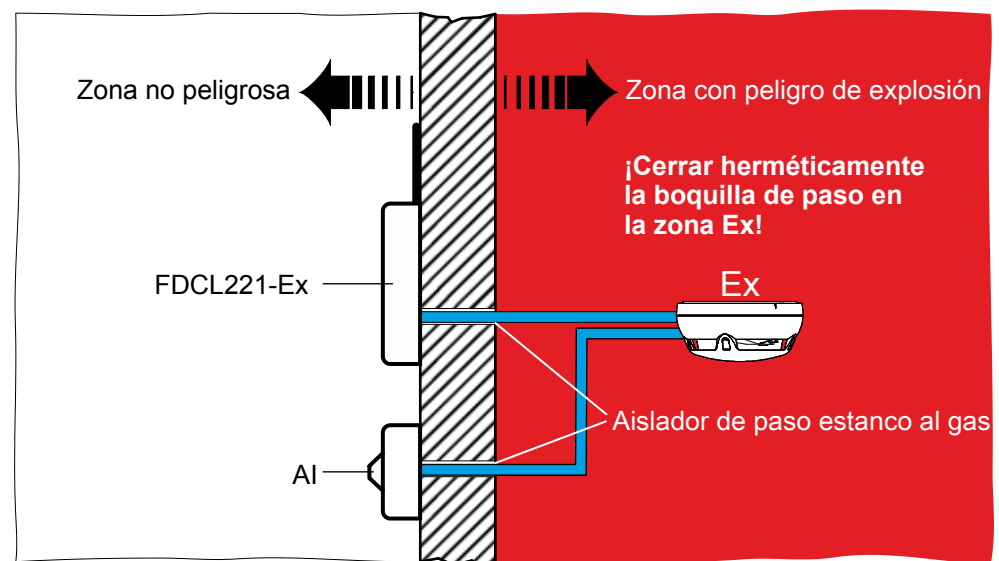
Figura 11: Representación esquemática de la disposición habitual de un indicador de alarma externo
