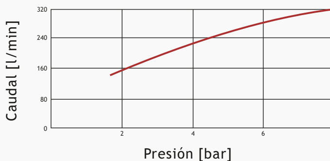
GRÁFICA CAUDAL / PRESIÓN
