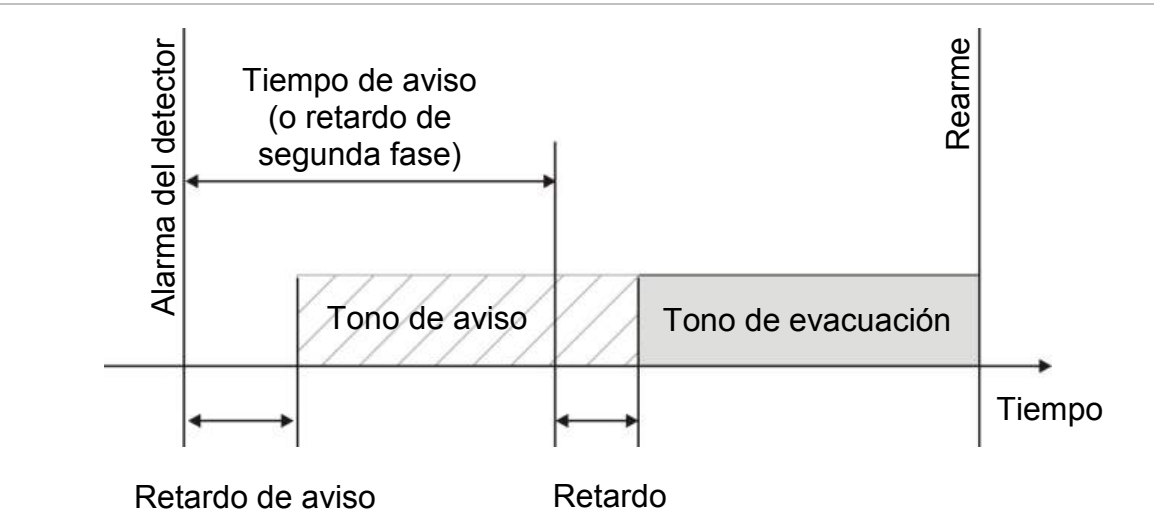
Figura 24: Alarma del detector con retardo de segunda fase
