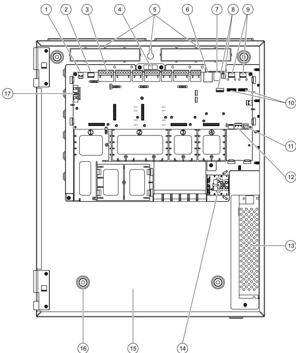
Figura 4: Diagrama del módulo grande y de la placa PCB (central de dos lazos)
