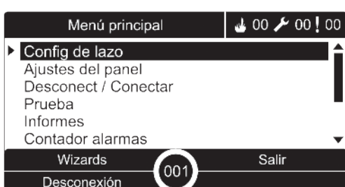
Figura 22: Menú principal del nivel de instalador
