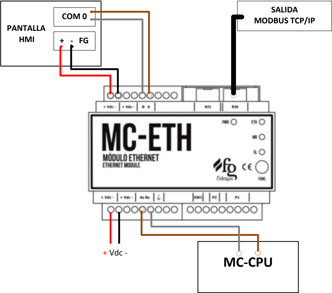
Imagen 17. Conexión con Módulo Ethernet MC-ETH-PMB.
