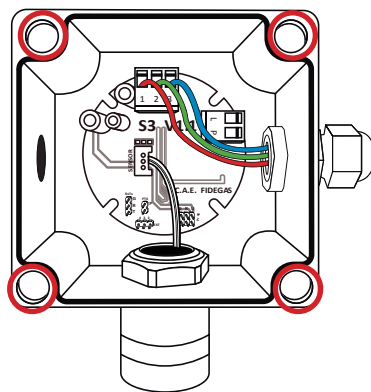
Instalación S/2-T2 ABS
