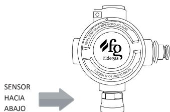
Figura 2: posición correcta de colocación del SRG
