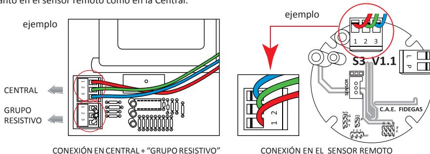
Figura 8: Conexión Central-Sensor remoto
