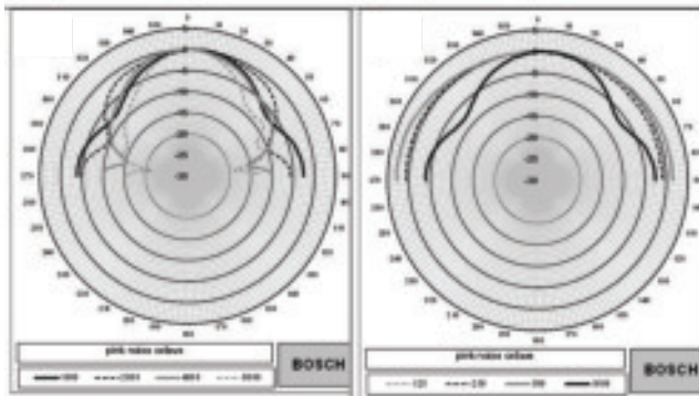
Diagramas polares
