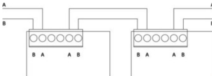
Figura 13: Conexiones de la tarjeta de red
