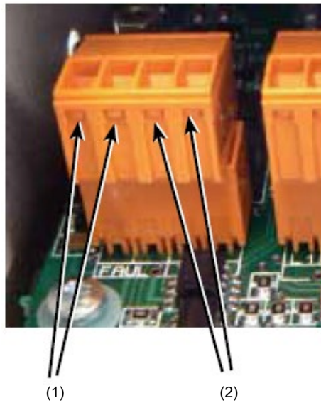
Figura 12: Contactos de relé Fault (Fallo) y Fire (Alarm) (Incendio (Alarma))
