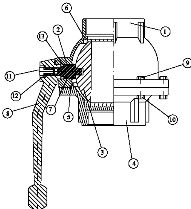
CONJUNTO LLAVE DE SECCIÓN E 1:2
