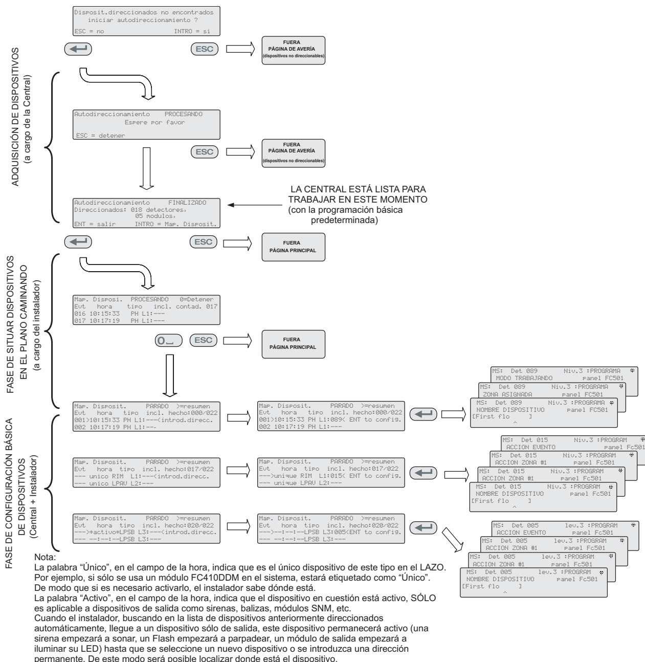
Figura 10 Procedimiento de Direccionamiento Automático
